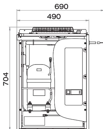
Внешний блок
