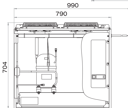
Внешний блок
